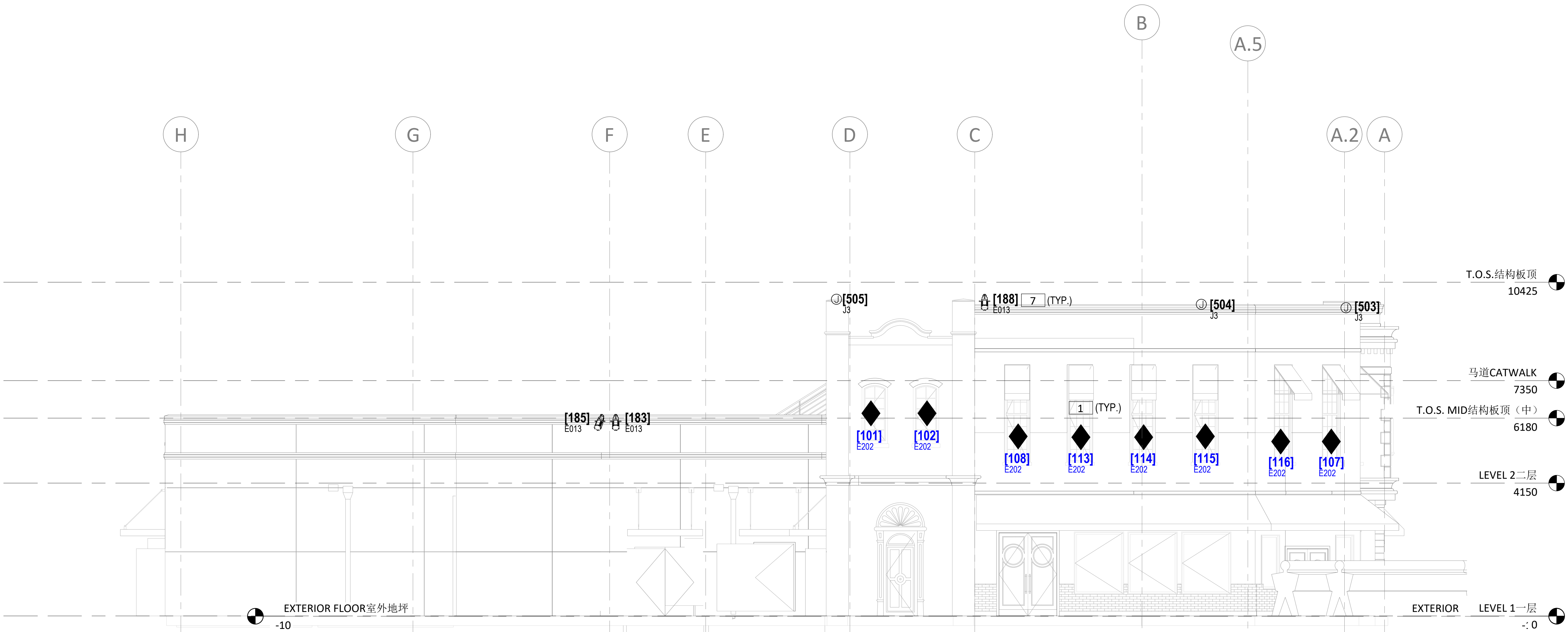
立面图 - 西 - 主题灯光 1 ELEVATION - WEST - THEMED LIGHTING TL201
